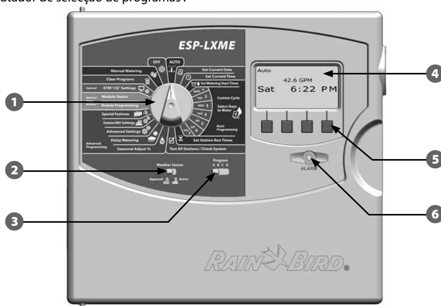
Funções do painel frontal do controlador ESP-LXME
