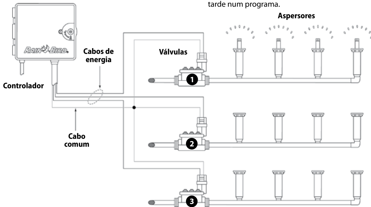
Esquema eléctrico do sistema LXME
